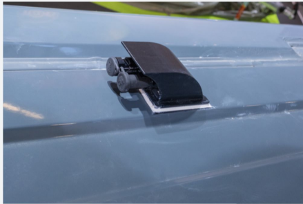
Plug-and-Play-Dachdurchführung für Solarmodule Geeignet für Solarstecker (MC4)
