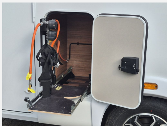
Gasflaschenauszug für max. 2 x 11 kg Gasflaschen
